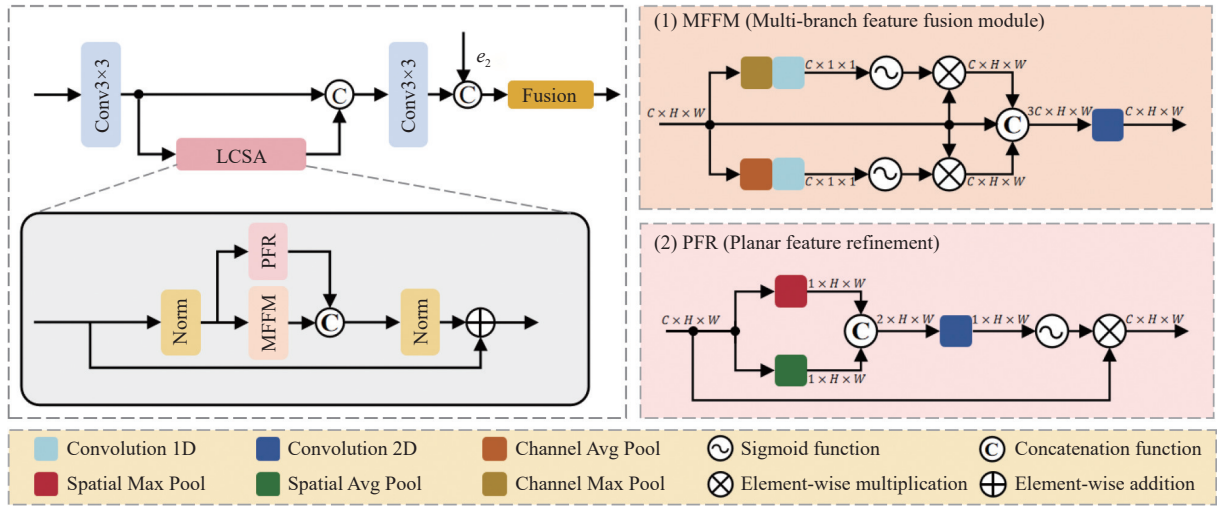
图 5 GA 编码器中 LCSA 模块的架构示意图
