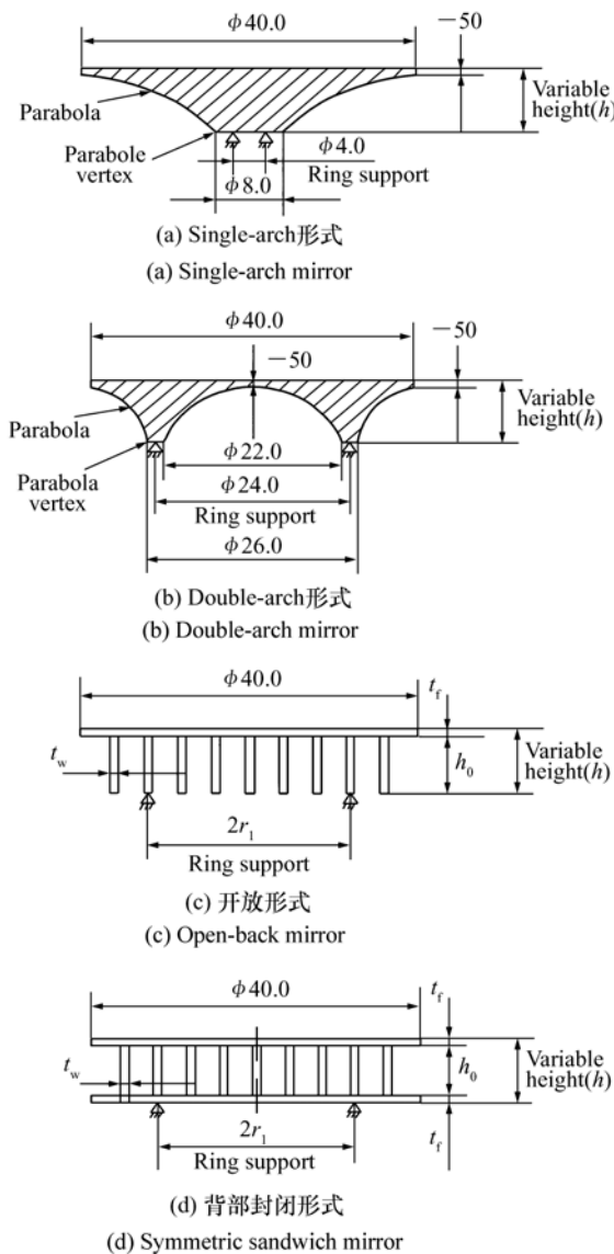
图1 反射镜轻量化结构示意图(单位:mm)
