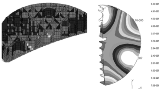
图 3 三角形孔优化
