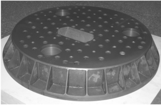
图5 实际的镜坯
